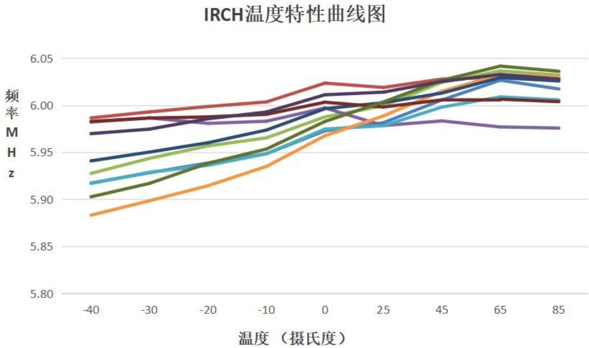
图 22-5-1 IRCH 温度特性曲线图
