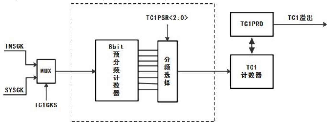
TC1 结构框图
