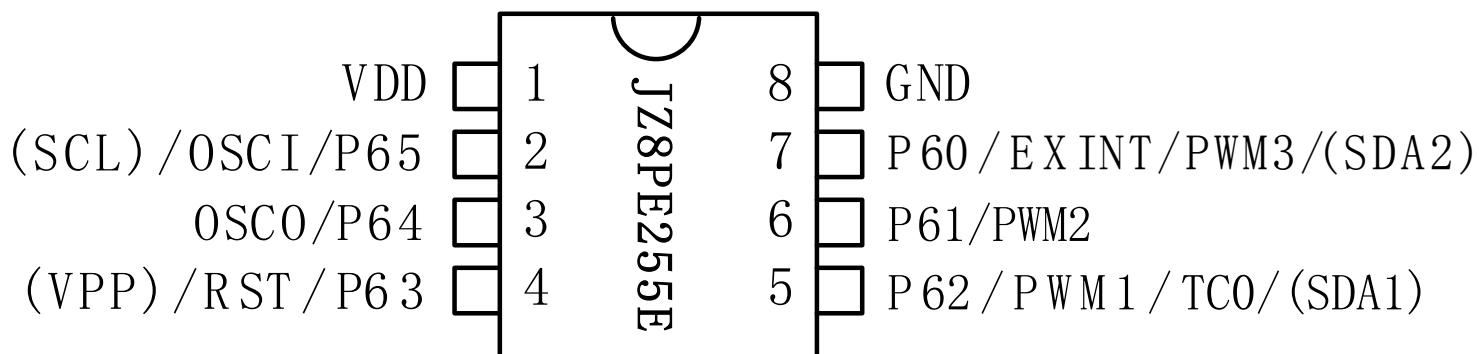
JZ8PE255E-8PIN 脚位图
