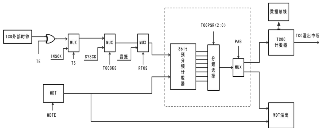
TC0/WDT 结构框图
