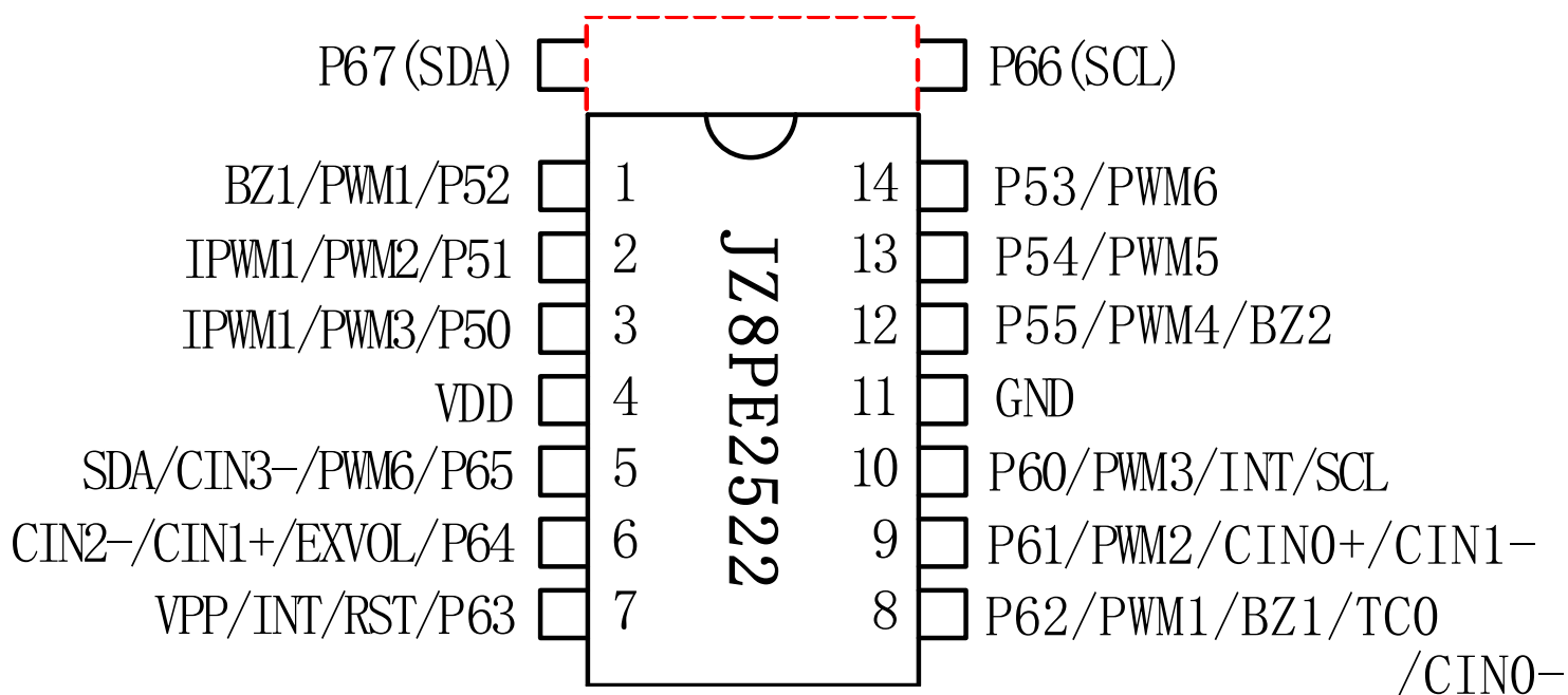
JZ8PE2522 - 14PIN 脚位图
