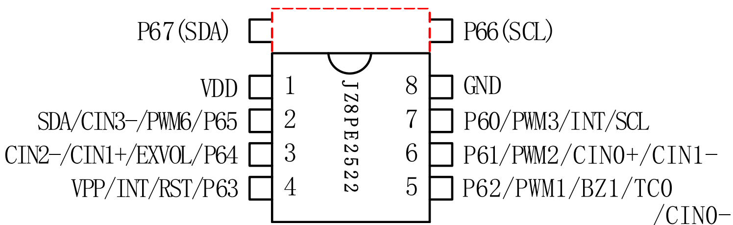
JZ8PE2522 - 8PIN 脚位图
