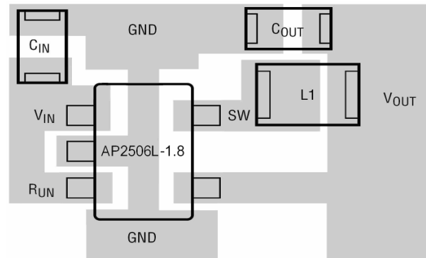
图 5. AP2506L 固定输出建议布局
