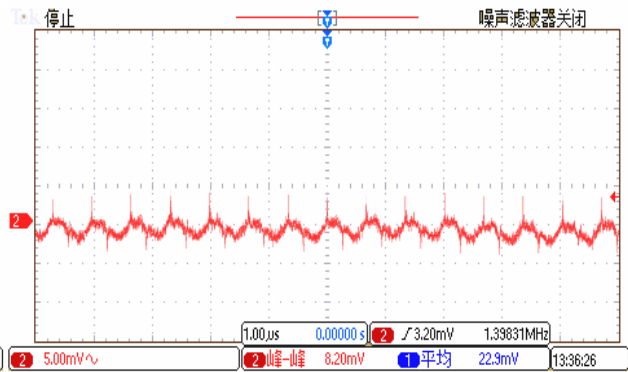
输出纹波
