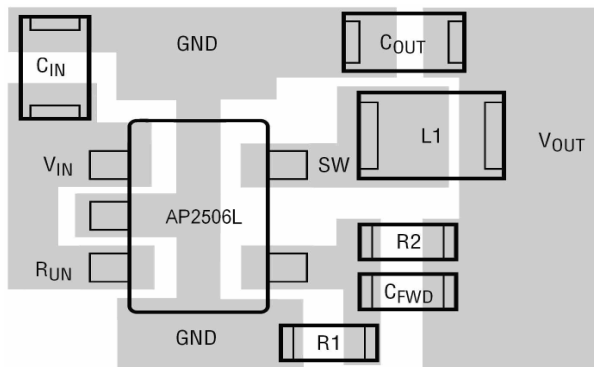
图 4. AP2506L 可调输出建议布局
