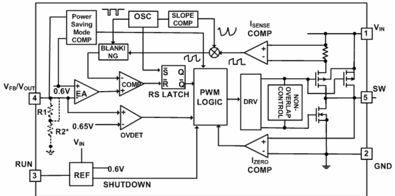
图 3 功能框图
